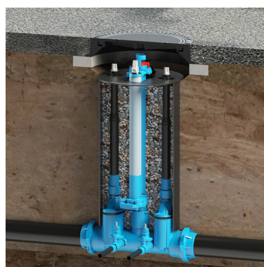
Einbausituation: Schalungsrohr mit Combi-III-Schieber
