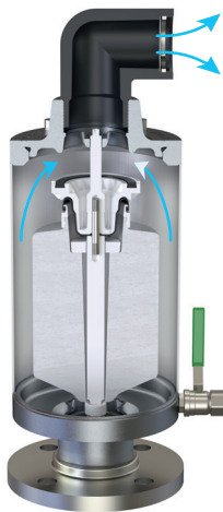
HaVent®: Anfahrventil Ventil offen
