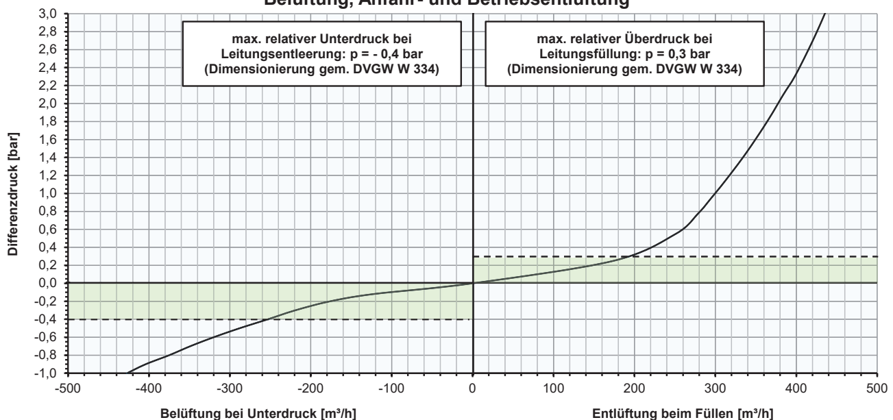
Leistungsdiagramm Be- und Entlüftungsventil Typ 986
