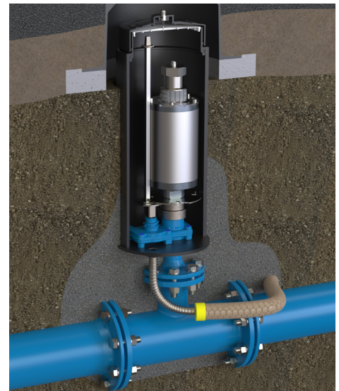
993-00 BEG aus PE mit HaVent®
