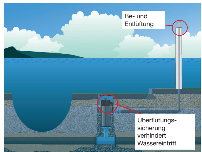
Einbausituation überflutet
