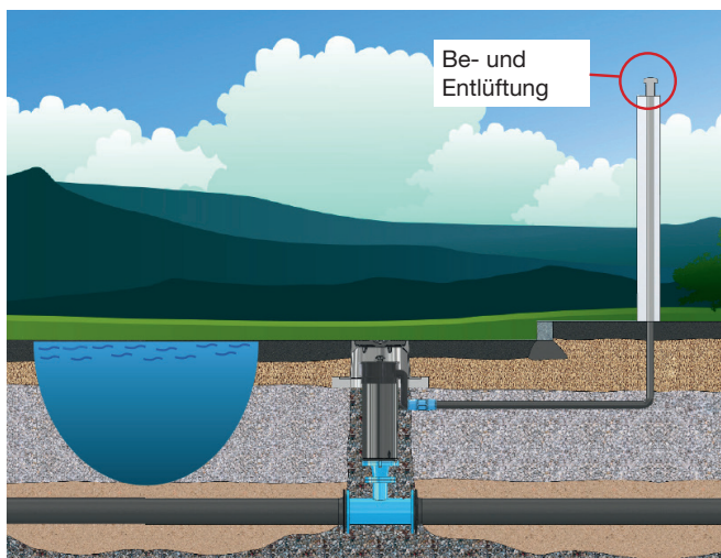
Einbausituation normal
