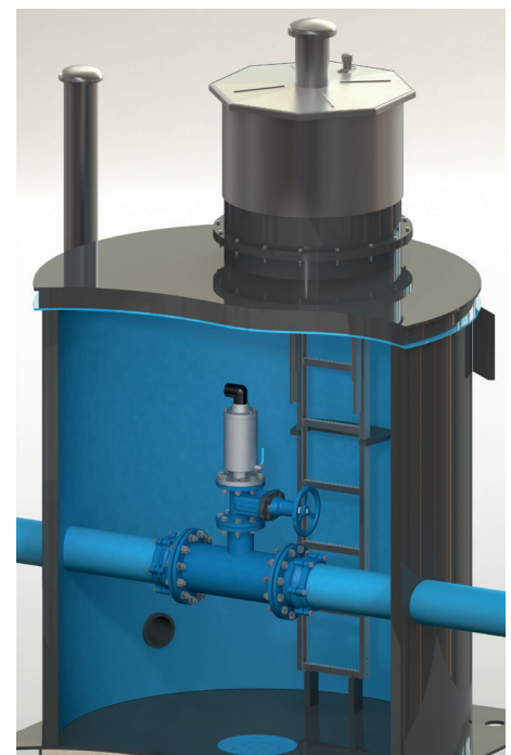
Hawle Armaturenschacht
