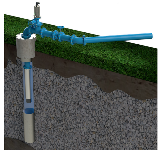
BEV HaVent® am Brunnenkopf
