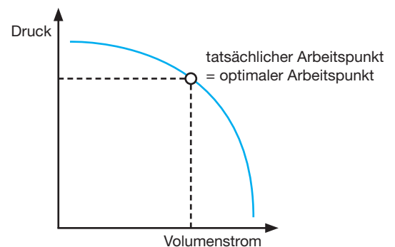
Rohrnetz mit BEV (Pumpenbetrieb)
