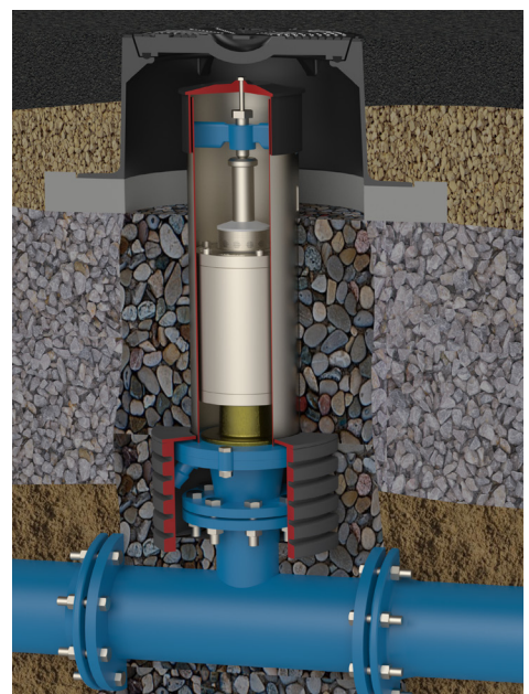
992-00 BEG aus nichtrostendem Stahl mit HaVent®
