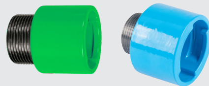
618-01 Übergangsstück mit ZAK® -Muffe und Außengewinde
