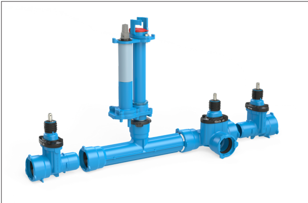
BAIO®-System: 5 Bauteile
