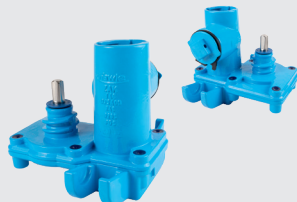
245-00 Universal-Hawlinger mit horizontaler ZAK®-Muffe 90° zur Rohrrichtung
