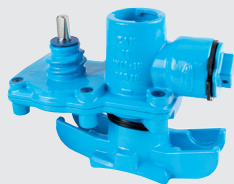
244-01 Universal-Hawlinger drehbar, mit horizontaler ZAK®-Muffe in Rohrrichtung
