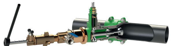
Anwendungsbeispiel im Abwasserbereich Anbohren einer Entsorgungsleitung durch Abwasser-Hausanschluss-Schieber ZAK 69 mit HAKU-Anbohrbrücke 45° (Best. Nr. 524-00) und Anbohrset ZAK69 45°
