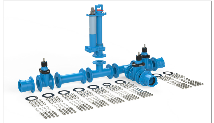
Flansch-System: 307 Bauteile
