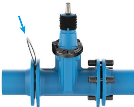
Einbau Schieber mit Festflanschen Problem: Einstecken der Dichtung
