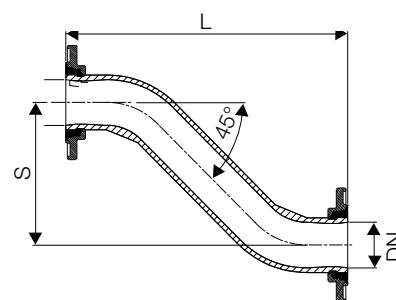
Ausführung Erdeinbau mit Einbaugarnitur
