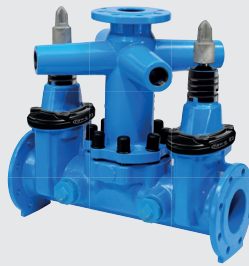
448-01 Combi-II-Schieber „WS/T“ mit FFR-Trommelstück
