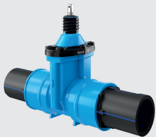
405-00 PE-Einschweiß-Schieber „E3“
