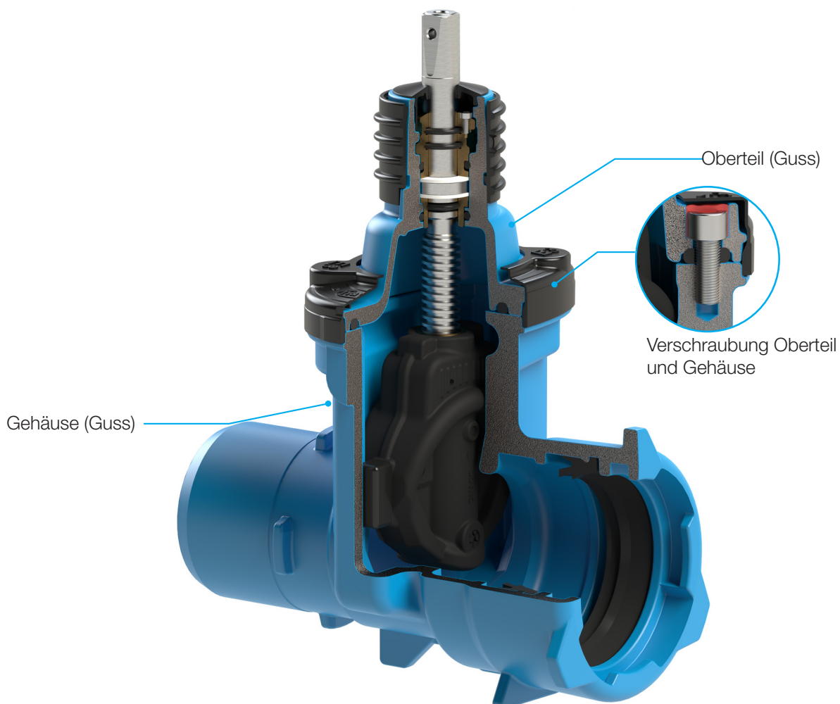
Abbildung: HSM-Schieber "E3", Best.-Nr. 451-00
