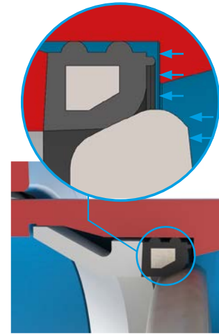
Funktionsprinzip 2 Klappenscheibe wird durch Betriebsdruck gegen Sitzdichtung gedrückt
