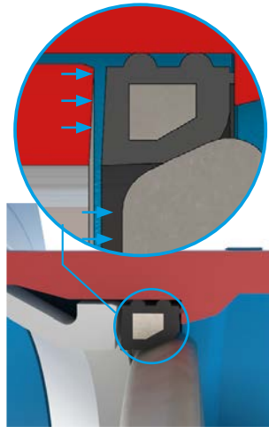
Funktionsprinzip 1 Sitzdichtung wird durch Betriebsdruck gegen Klappenscheibe gedrückt
