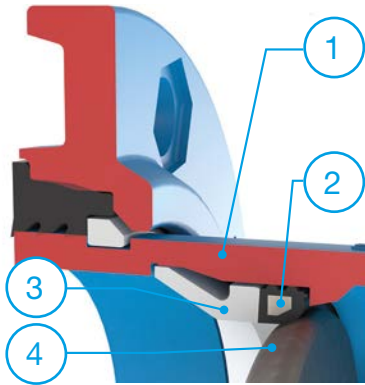
Schnittbild Dichtsystem
