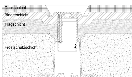
9. Kappe mit freigemachter Deckschicht
