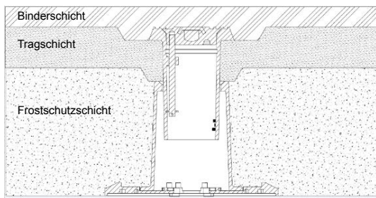
5. Kappe mit Binderschicht
