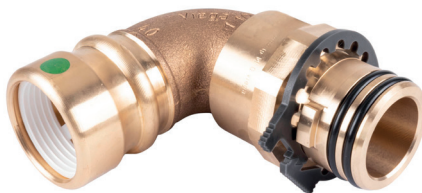
ZAK-Press-Fit®, Winkel 90° mit drehbarem Abgang Best.Nr. 647-05
