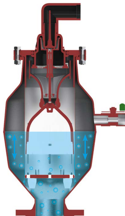
Abb.: Ventil geschlossen
