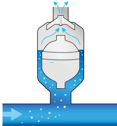
Aufgabe 2: Leitung im Betrieb: Betriebsventil
