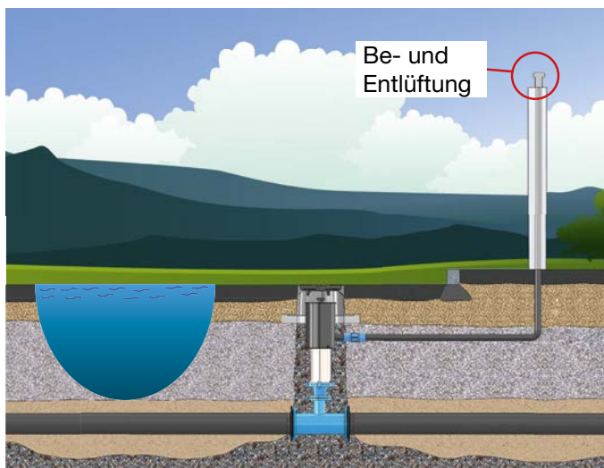
Einbausituation normal
