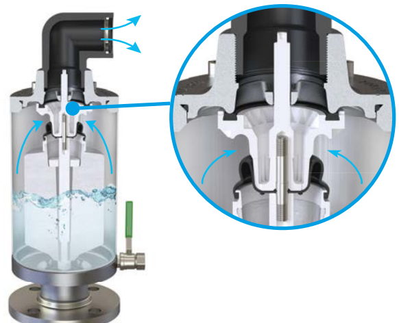
HaVent®: Betriebsentlüftung Rollmembran teilweise offen
