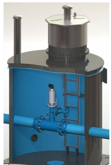
Hawle Armatureschacht
