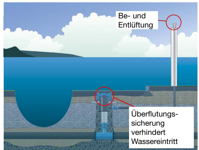
Einbausituation überflutet
