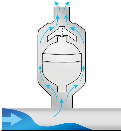
Aufgabe 1: Befüllung der Leitung: Anfahrventil
