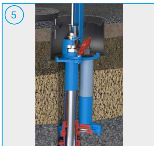
Aufsetzen des Einführwerkzeugs, anschließend den UFH unter vollem Betriebsdruck öffnen und finales Positionieren des Sensors in die Rohrleitung
