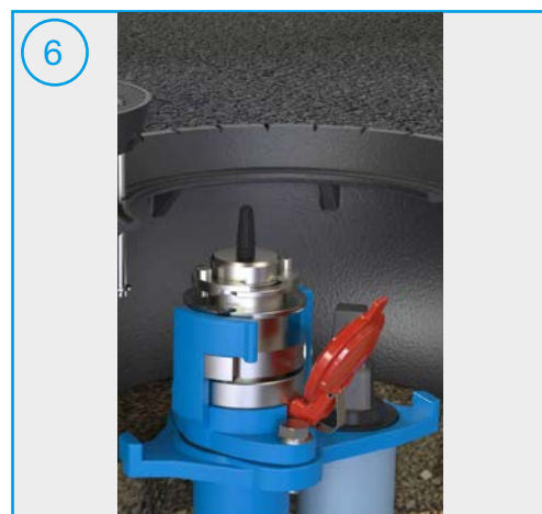
Montage der Sicherungsbleche, sowie der Antenne
