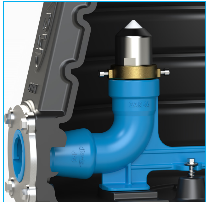
Abbildung: Einfache und schnelle Entnahme der Zählergarnitur durch das Hawle ZAK®-System. Reduzierte Schmutzanfälligkeit durch konische Bauweise.
